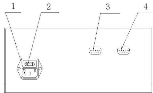
RK2511N 后面板示意图
