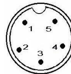
图 3.2.1：管脚排列图
